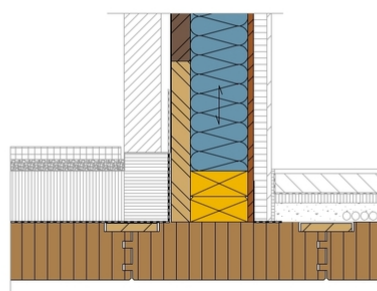
Anschluss Geschosdecke - Terrasse an Aussenwand
