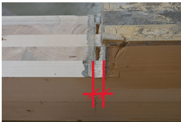
Comportement ductile de la came de cisailment en CLT sur l'éprouvette (lors des essais réalisés à l'ETH Zurich)
