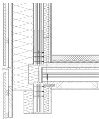
Détail du raccordement au plafond
