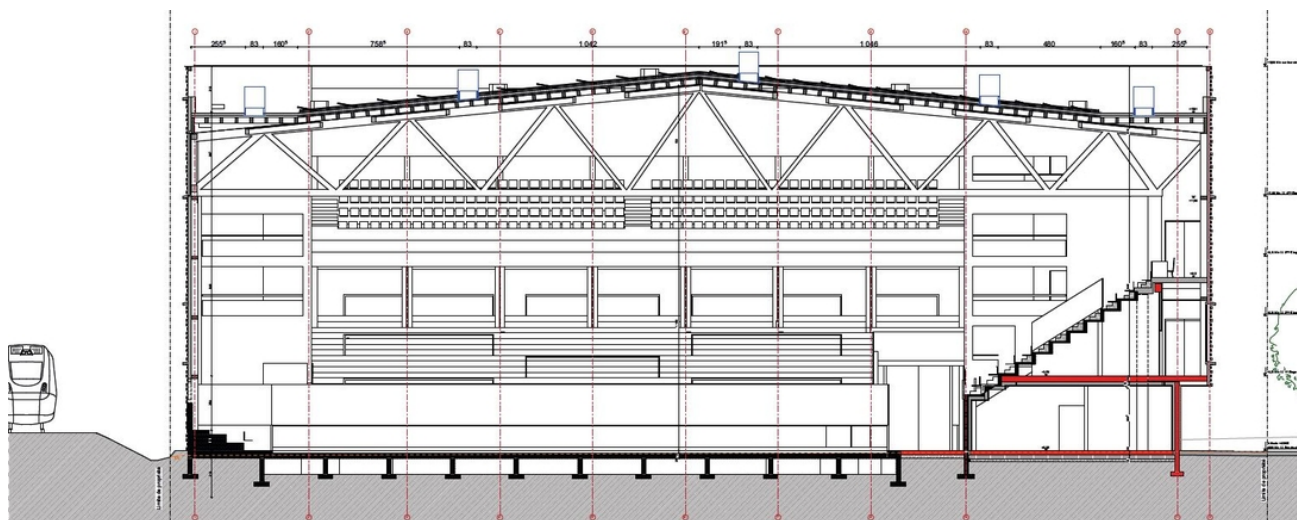
Coupe de la patinoire avec la charpente et la tribune en bois
