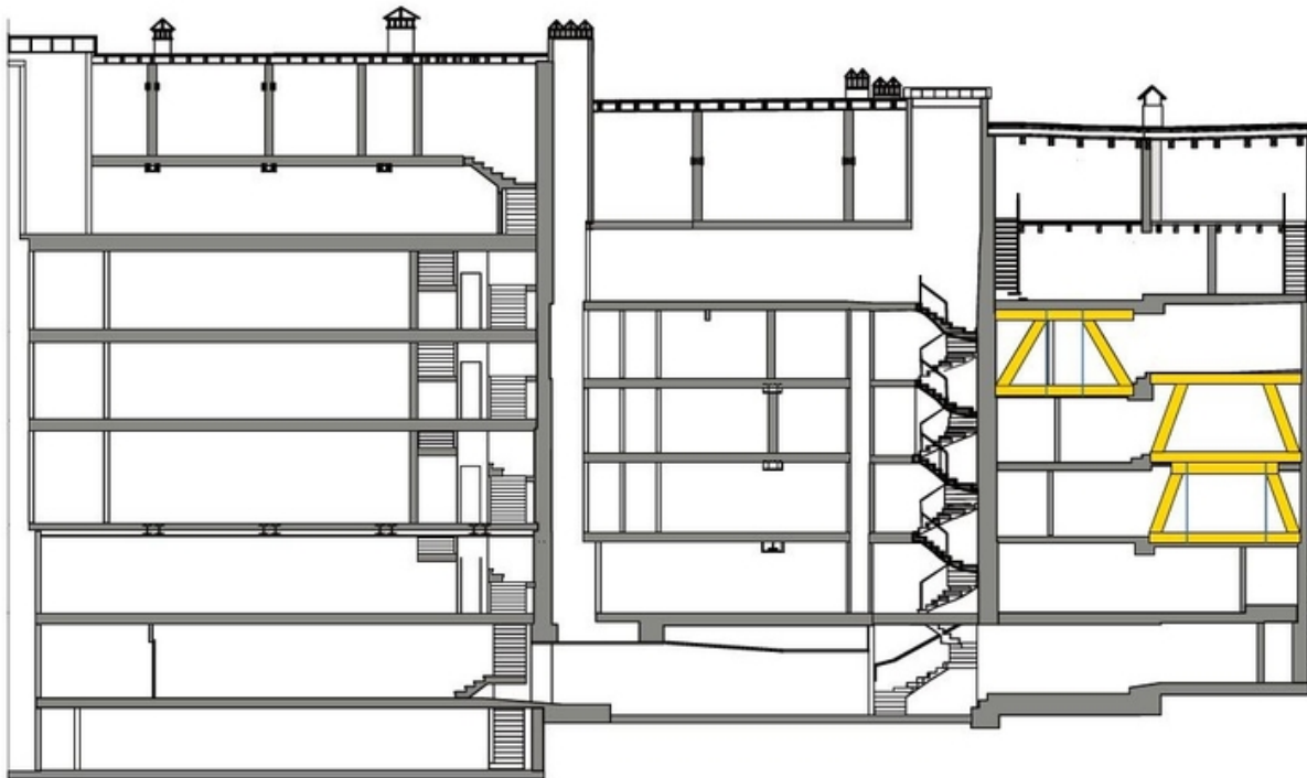
Des structures explosives en bois soutiennent les corps de bâtiments historiques.
