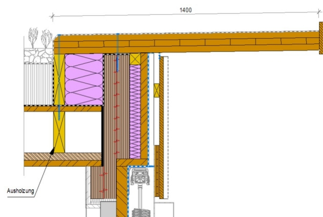
Detail Dachrand Abschluss
