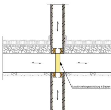
Detail Lastdurchleitung Wohnungstrennwand
