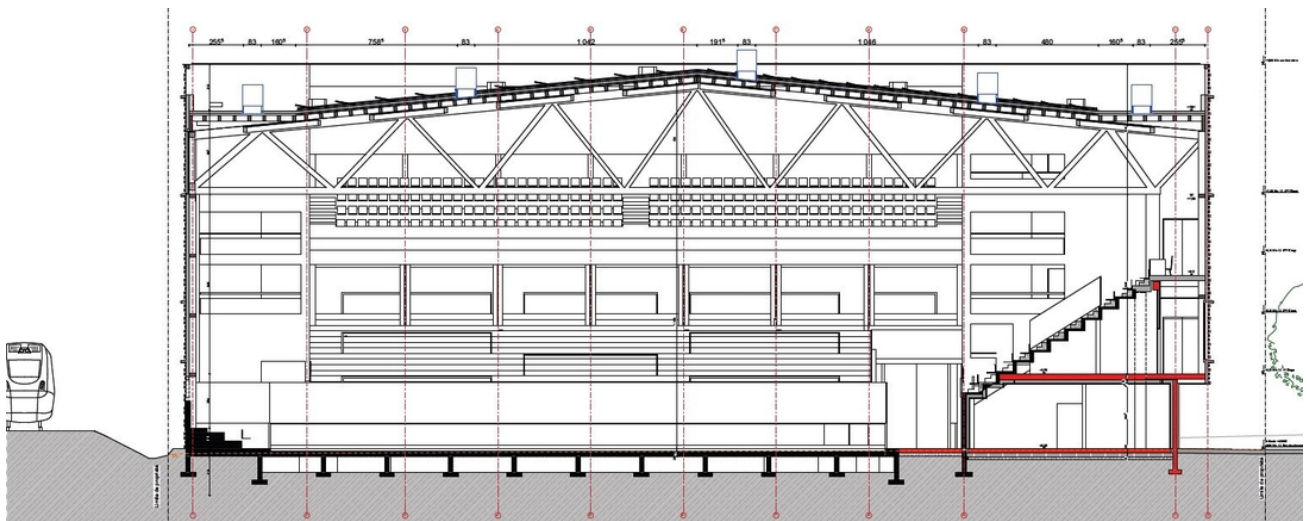
Schnitt durch die Eishalle mit dem Fachwerk und der Tribüne aus Holz
